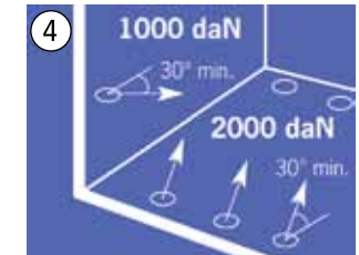
Panneau des points d'arrimage conformément à EN 12640 (dimensions minimales 200/150 mm)
