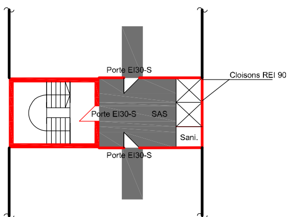
Figure 1: Ascenseur menant vers un étage avec bureaux paysagers ou bureaux combinés dans les bâtiments de type A.
